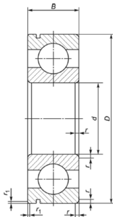
Рисунок 2 - Конструктивное исполнение 05
