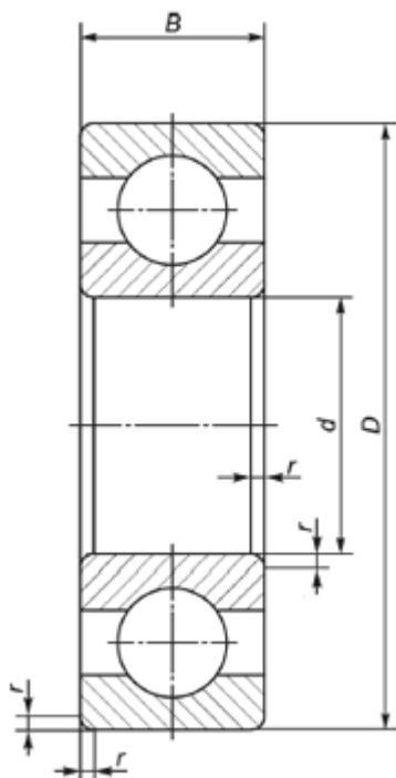
Рисунок 1 - Конструктивное исполнение 00
